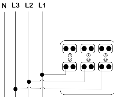
tropolni prekidač
