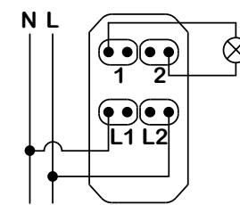
dvopolni prekidač
