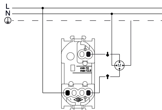
Prekidač za roletne
