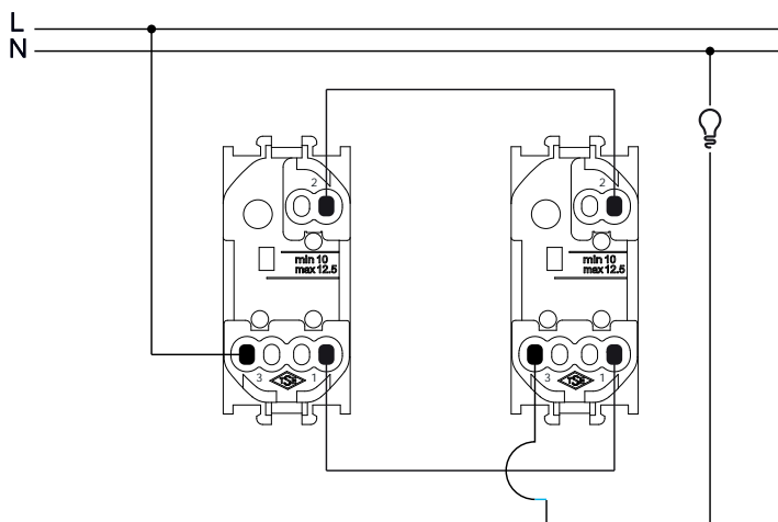
Dva dvopolna prekidača (s lokatorskom lampicom ili bez nje)
