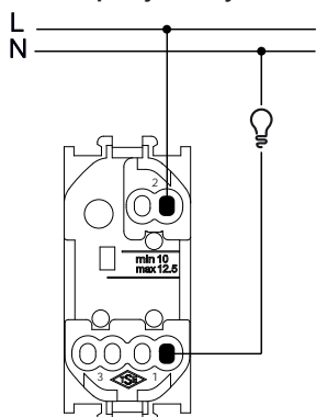
Jednopolni prekidač (s lokatorskom lampicom ili bez nje)
